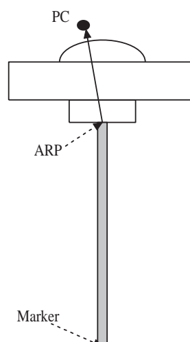
Figure 2-3: Antenna mount.
