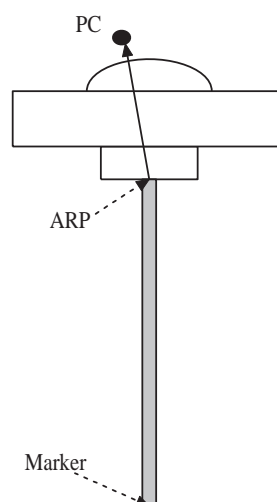
Figure 2-3: Antenna mount.
